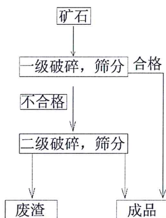
破碎工艺流程图
